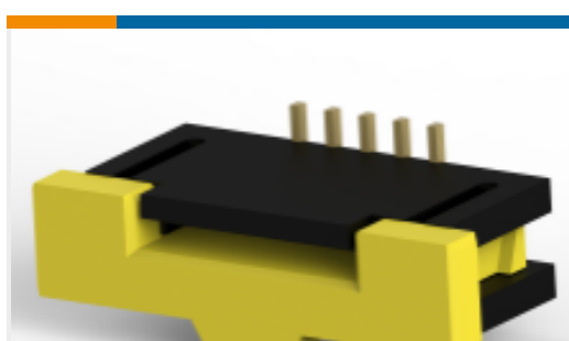
TE Part # 1734248-5 1.0 FPC, ZIF V/T, SMT, 5P
